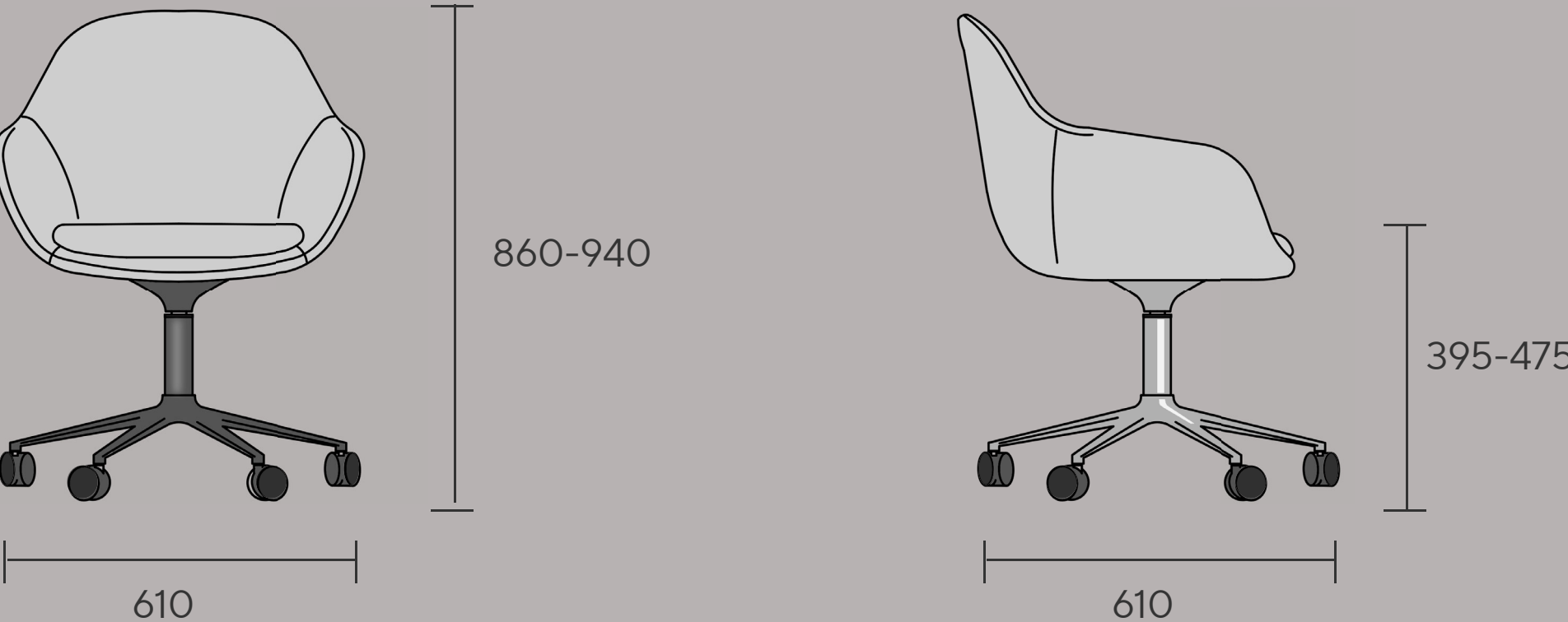
Кресло на колесах
